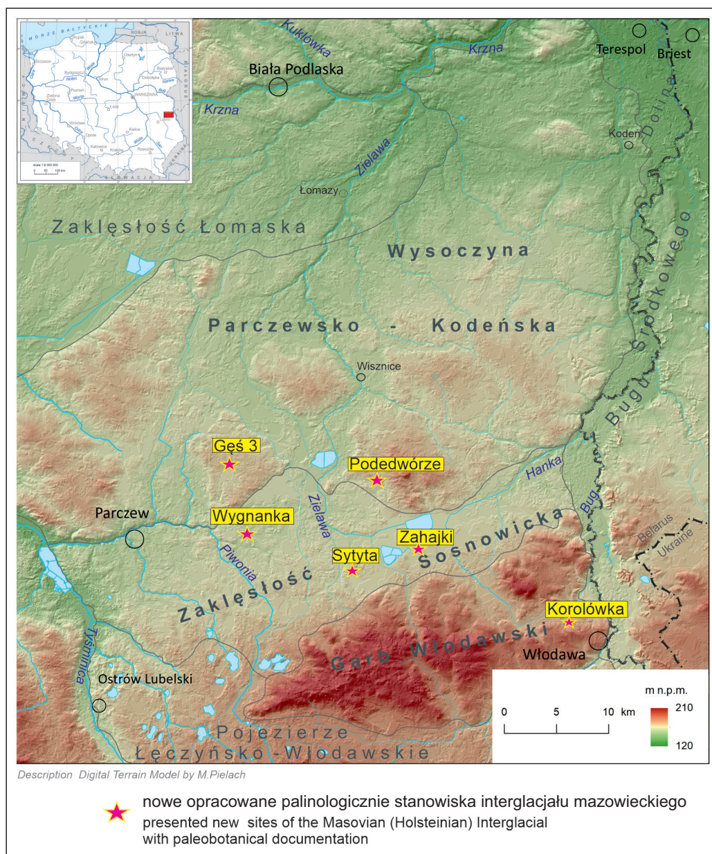
Fig. 1. Lokalizacja stanowisk z udokumentowanymi osadami interglacjału mazowieckiego na Zakłęstości Sosnowickiej i Garbie Włodawskim
