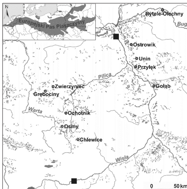
Fig. 1. Lokalizacja badanych stanowisk na tle rozmieszczenia pól wydymowych i większych pojedynczych wydym Fig. 1. Location of study sites against the distribution of dune fields and larger individual dunes
