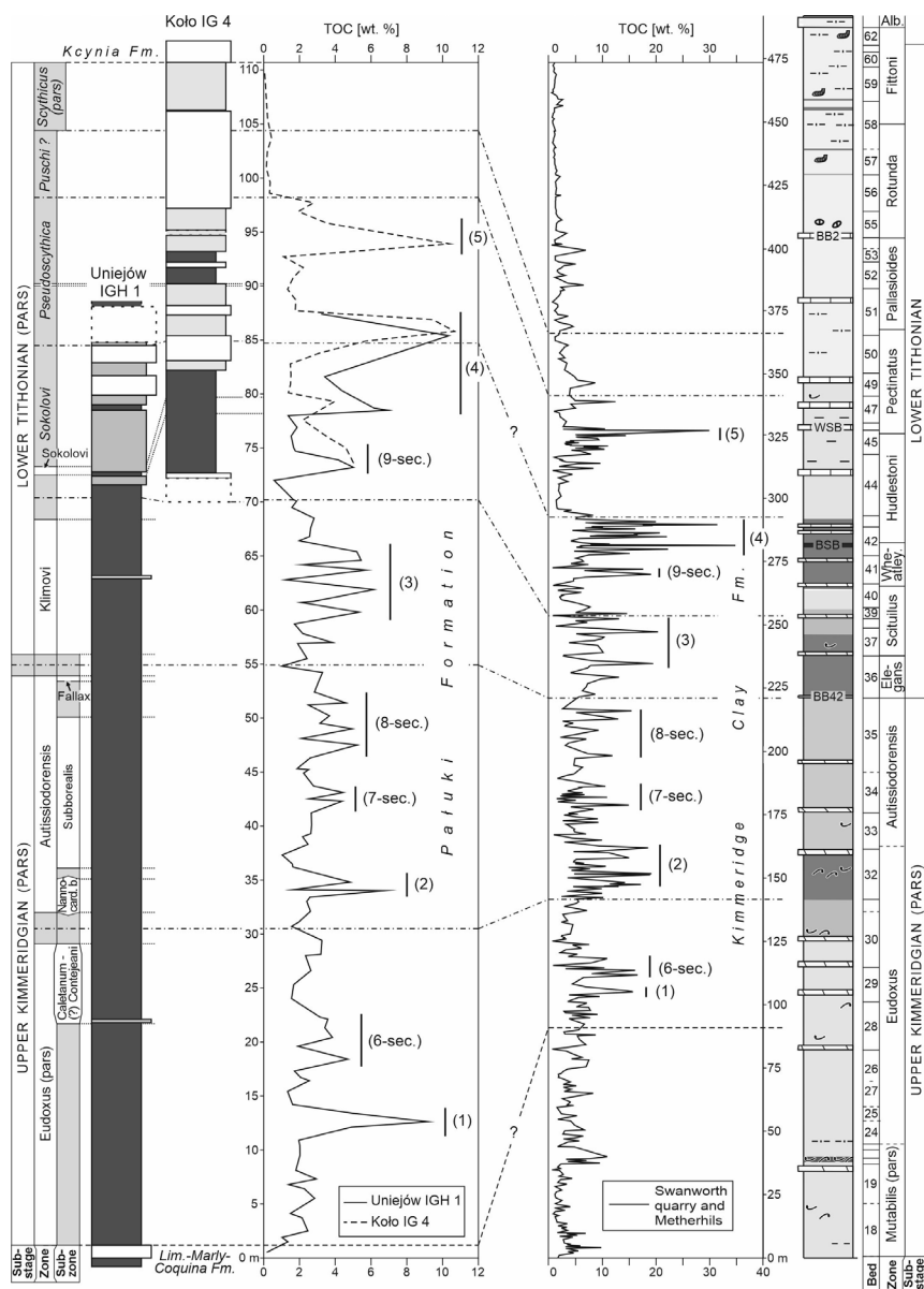
Fig. 1. Biostratigrafia i rozkład zawartości materii organicznej formacji pałuckiej oraz formacji Kimmeridge Clay (Morgans-Bell i in., 2001). Ścisła korelacja horyzontów wzbogaconych w materię organiczną jest prawdopodobnie związana z cyklami orbitalno-klimatycznymi
