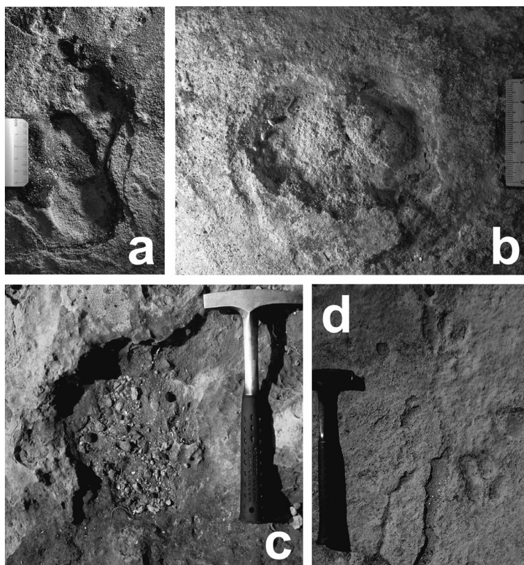
Fig. 1. Ichnoasocjacja z formacji Roka messynu zachodniej Krety: trop hominina z Trachilos (a); ślad przedstawiciela wołowatych z Falasarna (b); ślad słońia Proboscipeda isp. (c) i tropy małych nieparzystokopytnych (d) z Półwyspu Gramvousa
