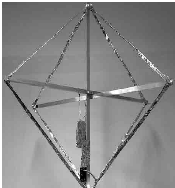
Antena detektora wraz ze wzmacniaczem. Przewody i wzmacniacz zostały owinięte folią aluminiową, aby zredukować zakłócenia pochodzące od urządzeń elektrycznych
