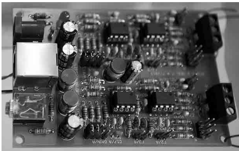
Wzmacniacz szerokopasmowy pozwala na wzmocnienie i wstępną obróbkę słabych impulsów elektrycznych zarejestrowanych przez antenę
