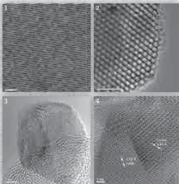
Obrazy z elektronowego mikroskopu transmisyjnego Titan 3 G2 60-300: (M. Rawski) 1. epitakcjonalna warstwa arsenku galu; 2. krzemionka SBA15; (G. Słowik) 3. krystalit PdZn w katalizatorze; 4. nanofaza tlenku kobaltu na powierzchni tlenku ceru
