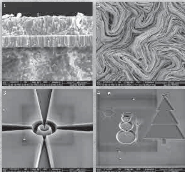
Obrazy z mikroskopu elektronowo-jonowego Quanta 3D FEG: 1. ceramika; 2. przekrój drutu miedzianego; 3. struktura spintroniczna; 4. test rozdzielczy FIB (M. Rawski, A. Brzyska)
