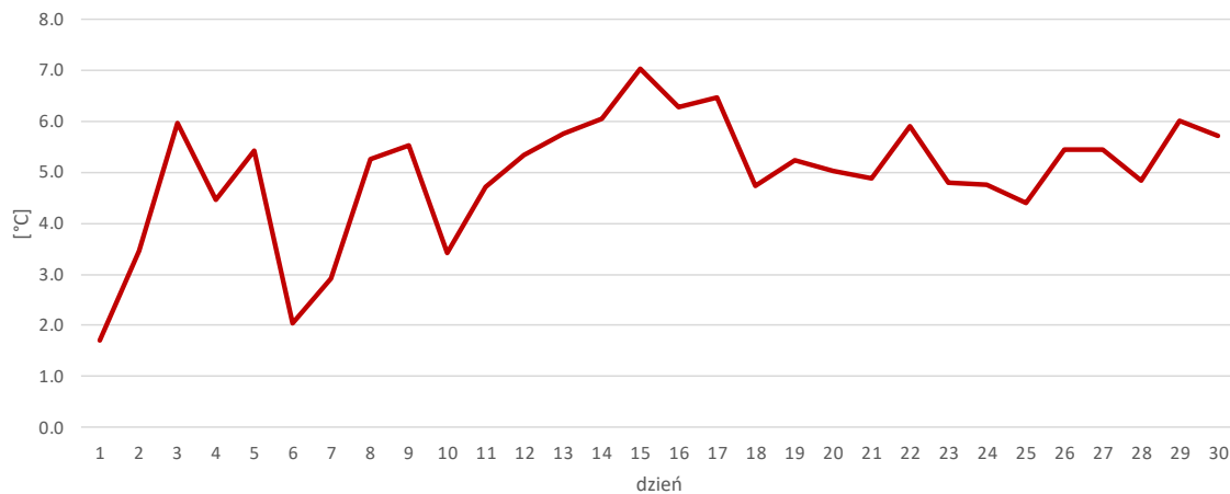
średnia dobowa temperatura powietrza - lipiec 2021
