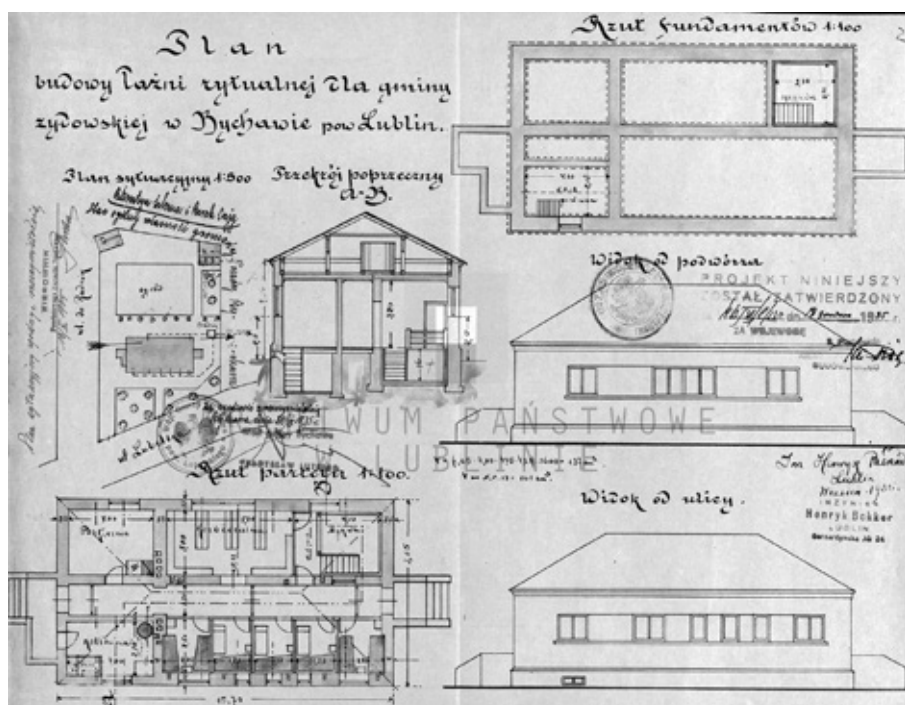
Ryc. 70. Plan budowy łaźni żydowskiej..., plan sytuacyjny, przekrój boczny (profil), rzut parteru, rzut fundamentów, rysunek elewacji tylnej, rysunek fasady. Źródło: APL. UWL. V WKB sygn.: 1673 k. 1–10 (www.szukajwarchiwach.pl)
