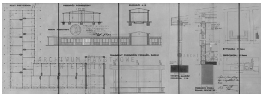
Ryc. 72. Projekt budek targowych w Bychawie, rzut przyziemia, przekrój poprzeczny, rysunek fasady, przekrój boczny (profil), fragment przekroju podłużnego, rysunek konstrukcji słupów, przekrój przez ścianę zewnętrzną, plan sytuacyjny, plan orientacyjny. Źródło: APL. UWL. V WKB sygn.: 1683 k. 1–5 ( www.szukajwarchiwach.pl )
