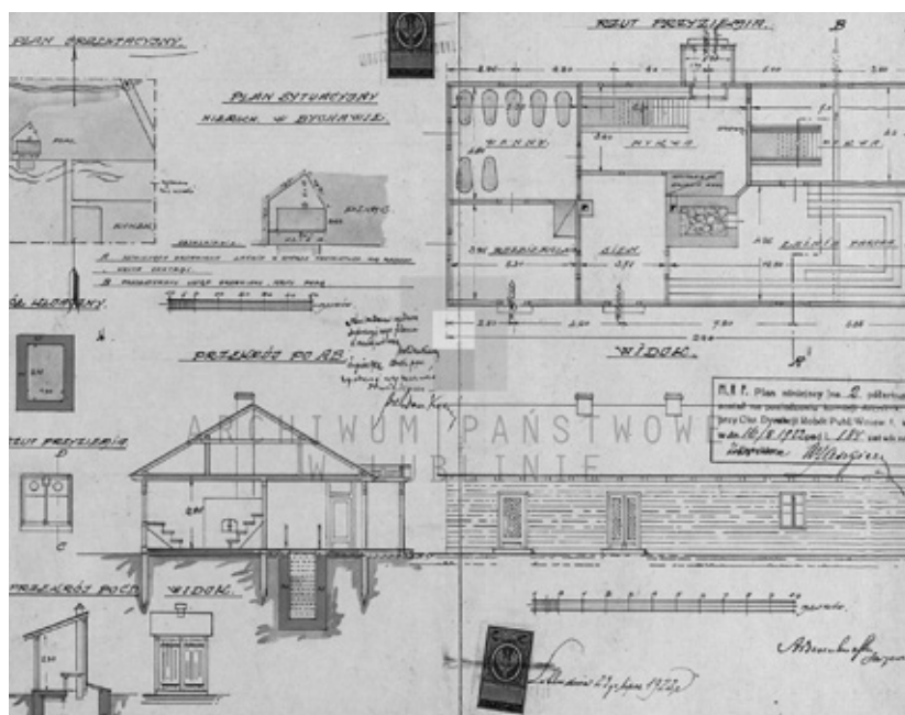
Ryc. 65. Plan przeróbki w drewnianej łaźni..., plan orientacyjny, plan sytuacyjny, rzuty wstępu, przekrój boczny (profil) mykwy, przekrój boczny i rysunek frontu wstępu, rzut mykwy, rysunek fasady mykwy. Źródło: APL. UWL. V WKB sygn.: 1672 k. 1–9 ( www.szukajwarchiwach.pl )
