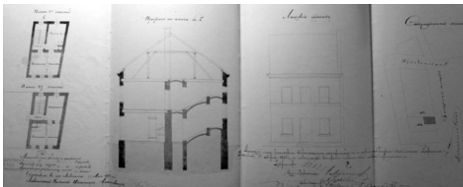
Ryc. 41. Plan domu nr 4... Rzut piętra, parteru, przekrój boczny, fasada, plan działki. Źródło: APL. RGL. B I sygn.: 1892:10 k. 25, fot. autor
