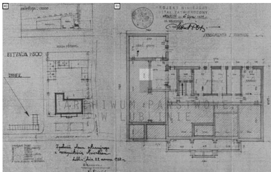
Ryc. 71. Projekt Zarządu Gminnego w Bychawie, plan orientacyjny, plan sytuacyjny, rzut fundamentów. Źródło: APL. UWL. V WKB sygn.: 1677 k. 1–12 ( www.szukajwarchiwach.pl )
