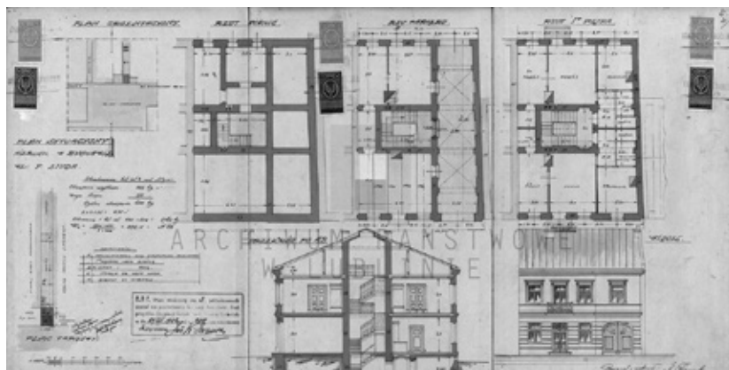
Ryc. 64. Plan domu nr 20..., plan orientacyjny, plan sytuacyjny, rzut poziomy piwnic, rzut parteru, przekrój ściany bocznej (profil), rzut piętra, rysunek fasady. Źródło: APL. UWL. V WKB sygn.: 1687 k. 1–7 ( www.szukajwarchiwach.pl )
