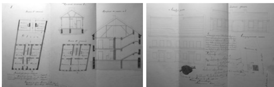
Ryc. 40. Plan domu nr 3... a) Rzut parteru domu i stodoły, profil stodoły, rzut piętra domu, profil domu; b) Fasada domu, fasada stodoły, plan działki. Źródło: APL. RGL. B I sygn.: 1892:10 k. 19-20, fot. autor
