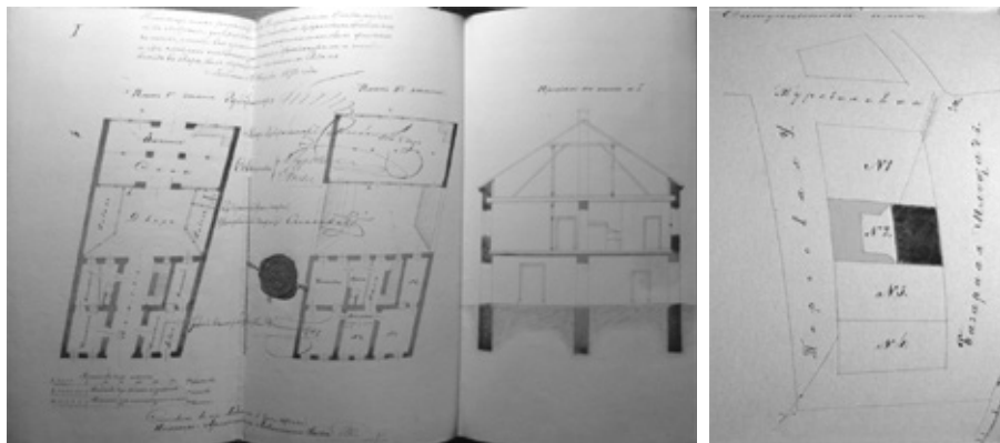
Ryc. 39. Plan domu nr 2... a) Rzut parteru, piętra, przekrój boczny; b) Plan działki. Źródło: APL. RGL. B I sygn.: 1892:10 k. 29-30, fot. autor
