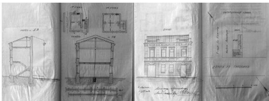
Ryc. 57. Projekt domu nr 63... Profil AB, rzut parteru, rzut piętra, profil CD, rysunek fasady, plan sytuacyjny. Źródło: APL. RGL. B I sygn.: 1908:7 k. 12–15, fot. autor
