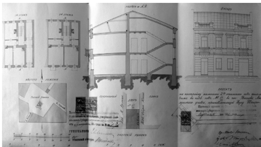
Ryc. 61. Projekt domu nr 64... Rzut parteru, rzut piętra, plan orientacyjny, profil budynku, plan sytuacyjny, rysunek fasady. Źródło: APL. RGL. B I sygn.: 1911, fot. autor
