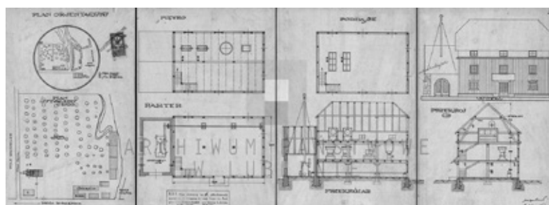
Ryc. 68. Projekt młyna P. Kryski... , plan orientacyjny, plan sytuacyjny, rzut piętra, rzut parteru, rzut poddasza, przekrój poprzeczny, rysunek fasady, przekrój boczny (profil). Źródło: APL. UWL. WKB sygn.: 1543 k. 1–7 ( www.szukajwarchiwach.pl )
