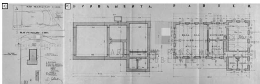
Ryc. 69. Projekt rzeźni w Bychawie, plan orientacyjny, plan sytuacyjny, rzut fundamentów, rzut parteru. Źródło: APL. UWL. V WKB sygn.: 1594 k. 1–8 (www.szukajwarchiwach.pl)
