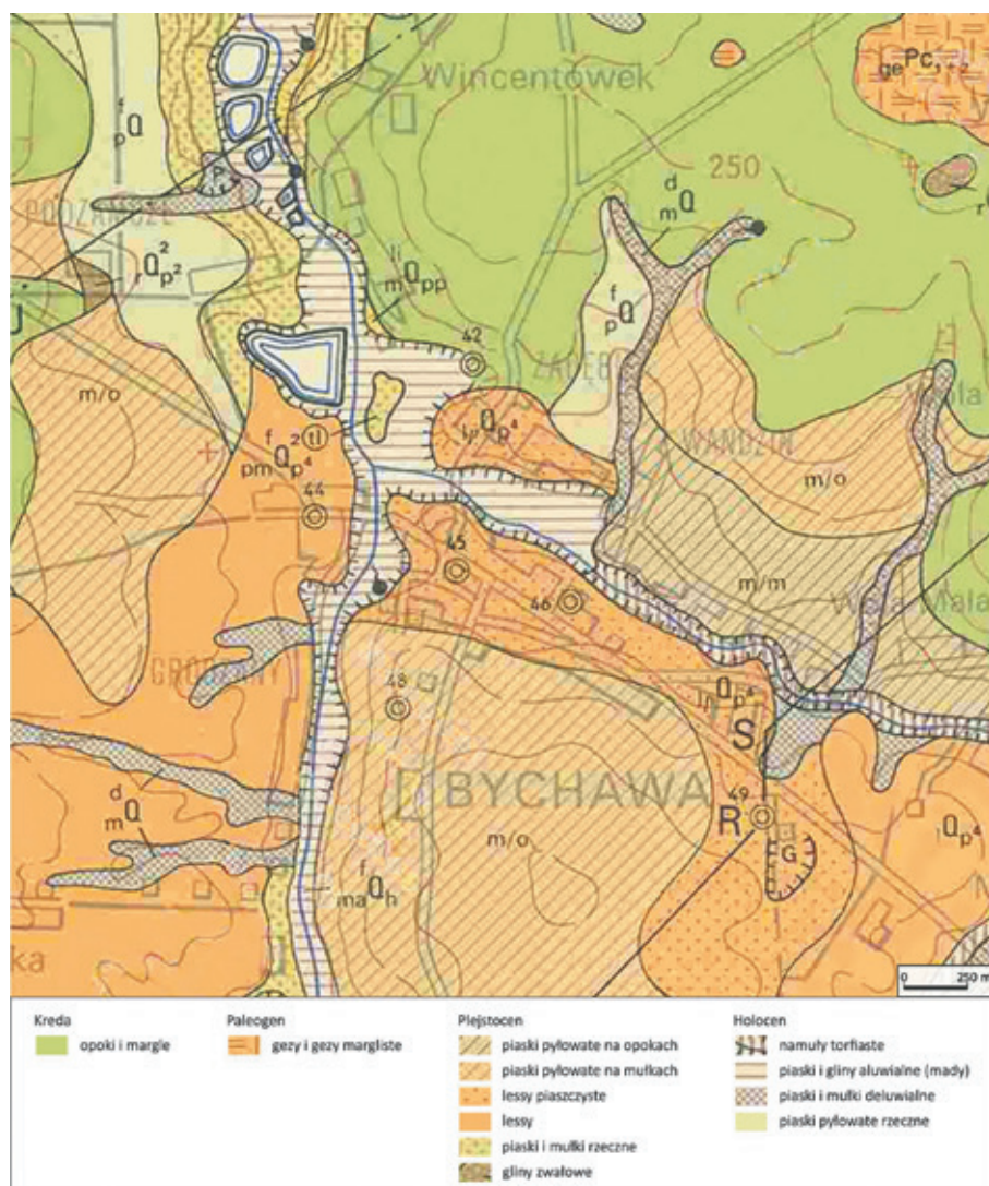
Ryc. 4. Utwory powierzchniowe w okolicy miasta Bychawa.
