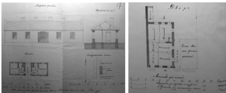
Ryc. 46. Plan domu W. Korony... Fasada, rzut parteru, profil, plan działki. Źródło: APL. RGL. B I sygn.: 1892:10 k. 16–17, fot. autor
