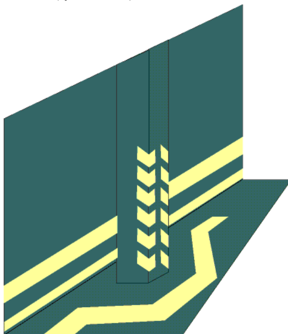
Rys. 22. Przykład oznakowania przeszkód na drodze ewakuacyjnej.
