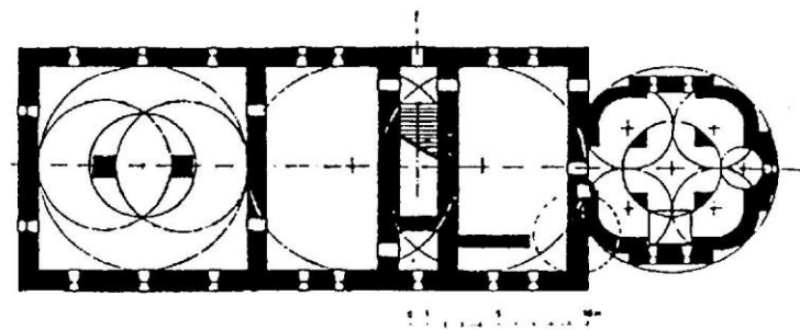
Rys. 35. Ostrów Lednicki. Plany i próby rekonstrukcji dwu faz założenia kaplica-palatium. Oprac. T. Węclawowicz. Wg Żurowska i in. 1993.
