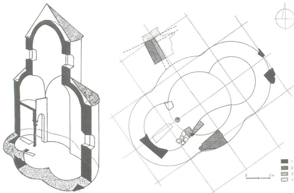
Ryc. 12. Kościół B. Rekonstrukcja bryły budowli według S. Koziela oraz schemat modułowy trzeciej fazy kościoła B w postaci dwuabsydowej rotundy z emporą zachodnią i dwoma aneksami zewnętrznymi według S. Koziela i M. Frasia. 1 – mury pierwszej fazy; 2 – mury drugiej fazy; 3 – mury trzeciej fazy; 4 – wylewka na zewnątrz i we wnętrzu aneksu b.
