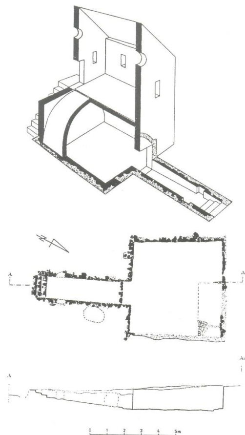
Ryc. 7. Budowla czworokątna. Plan odsłoniętych reliktów budowli czworokątnej z korytarzem według A. Żakiego oraz próba rekonstrukcji budowli według Z. Pianowskiego.
