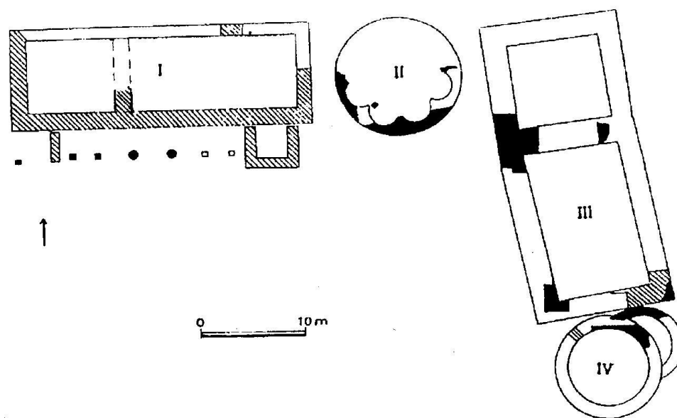
Rys. 32. Wiślica. Romańskie budowle na „regii”. Wg Wartołowska (uzupełnienia wg Gliński).
