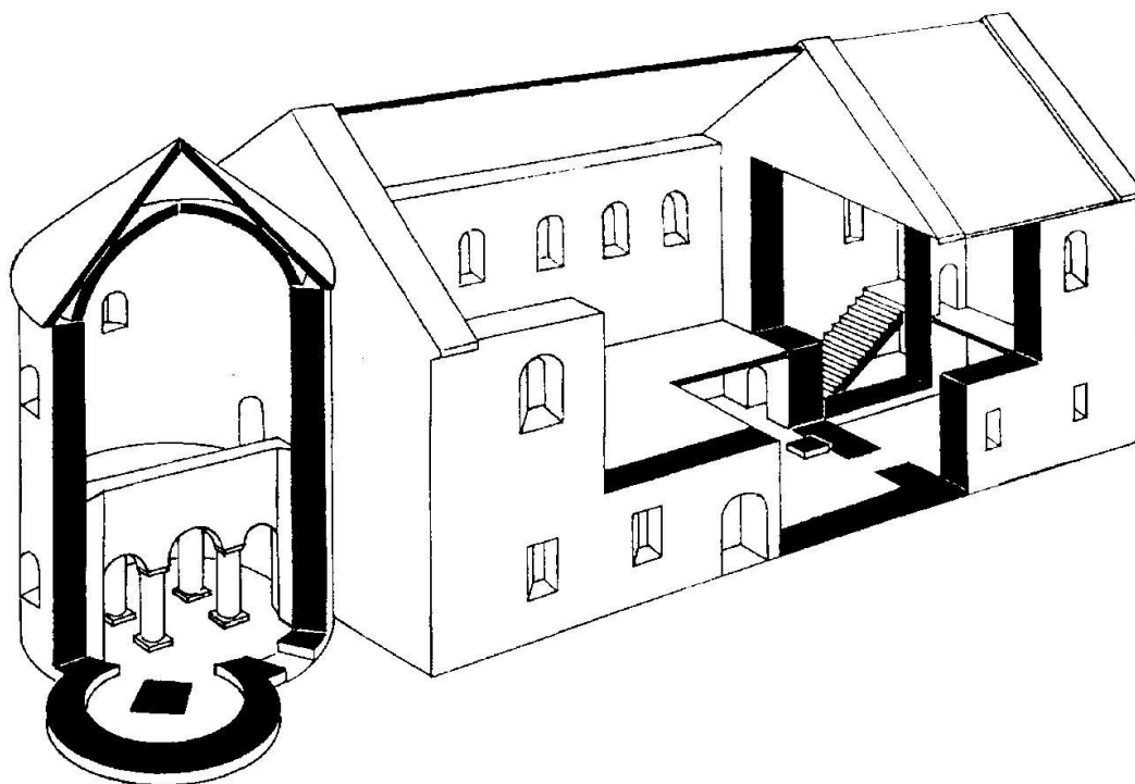
Rys. 20. Próba aksonometrycznej rekonstrukcji zespołu rotunda-palatium wg stanu
