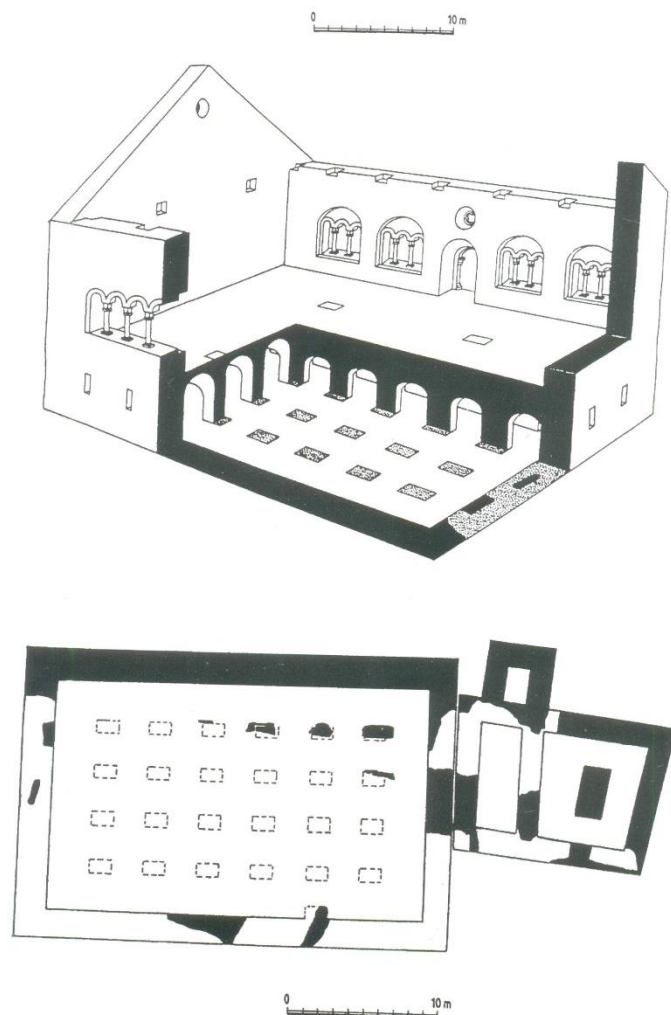
Ryc. 27. Sala o 24 słupach. Rekonstrukcja planu z zaznaczeniem odkrytych reliktów rzymskiego palatium i aneksu kaplicy po badaniach A. Szyszko-Bohusza, J. Firleta i Z. Pianowskiego oraz rekonstrukcja bryły rzymskiego palatium według Z. Pianowskiego. Przekrój aksometryczny.
