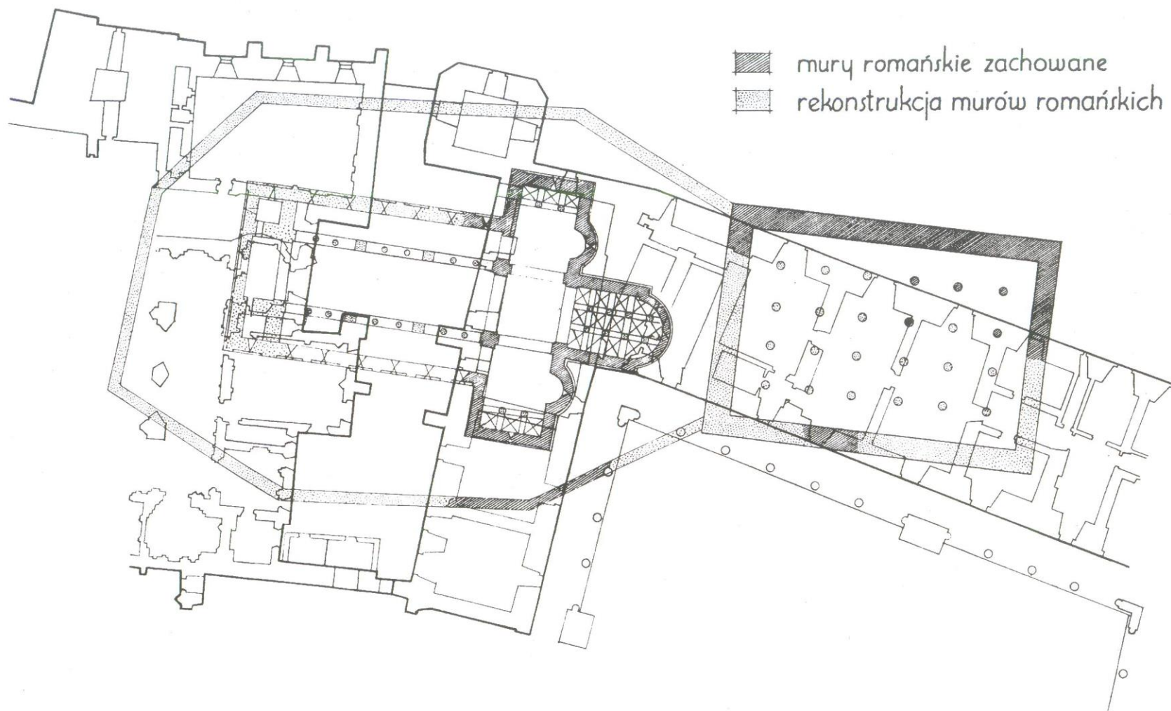
Ryc. 25. Bazylika tzw. św. Gereona. Rekonstrukcja tzw. pierwszej katedry romańskiej oraz sali o 24 słupach według A. Szysko-Bohusza.
