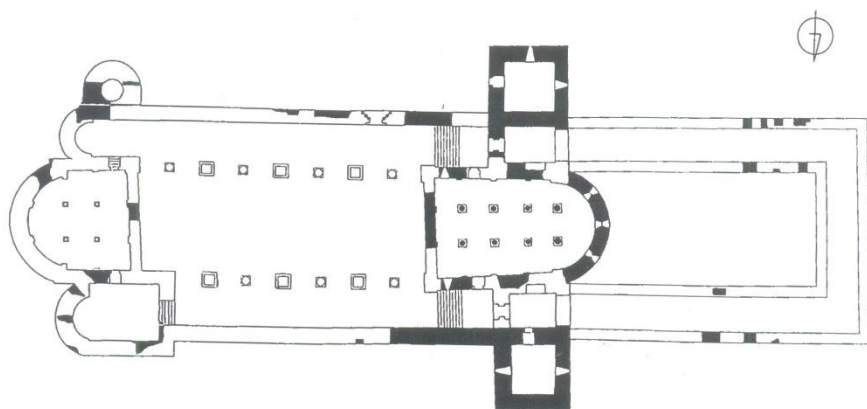
Ryc. 20. Katedra romańska. Rekonstrukcja planu katedry romańskiej po badaniach S. Odrzywolskiego, A. Szyszko-Bohusza, J. Firleta i Z. Pianowskiego oraz rekonstrukcja kościoła katedralnego według Z. Pianowskiego. Przekrój aksonometryczny.
