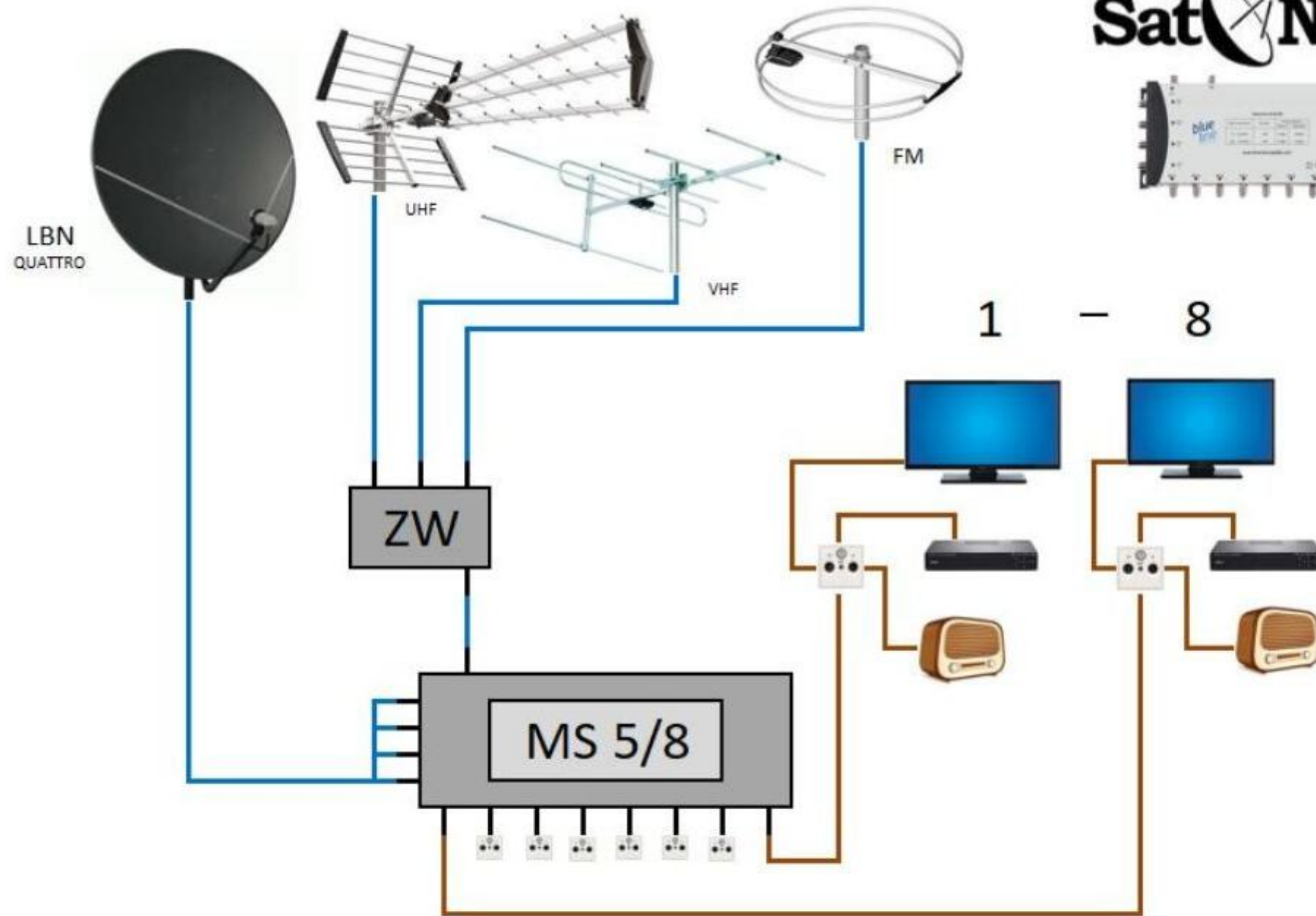
Tradycyjna instalacja zbiorcza SAT-TV-R dla domu jednorodzinnego z wykorzystaniem jednego satelity.
