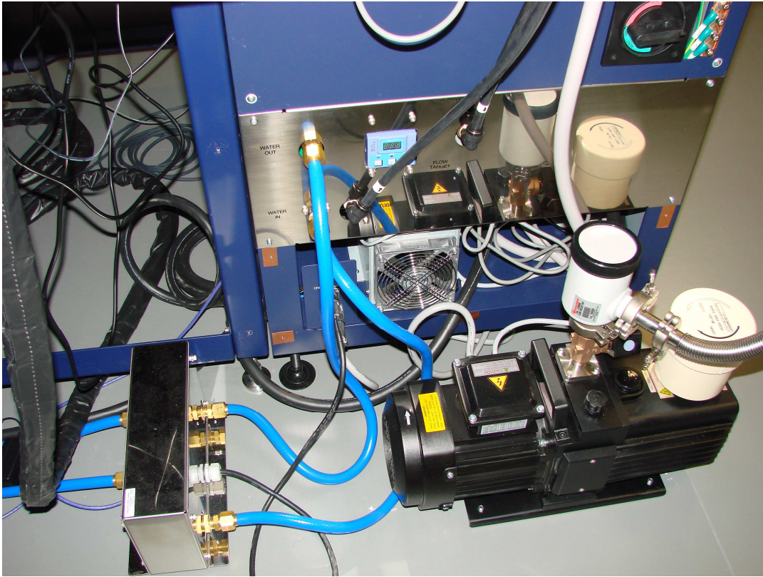
OPTYKA OGNISKUJĄCA WIĄZKĘ (Z POMPĄ PRÓŻNIOWĄ)
