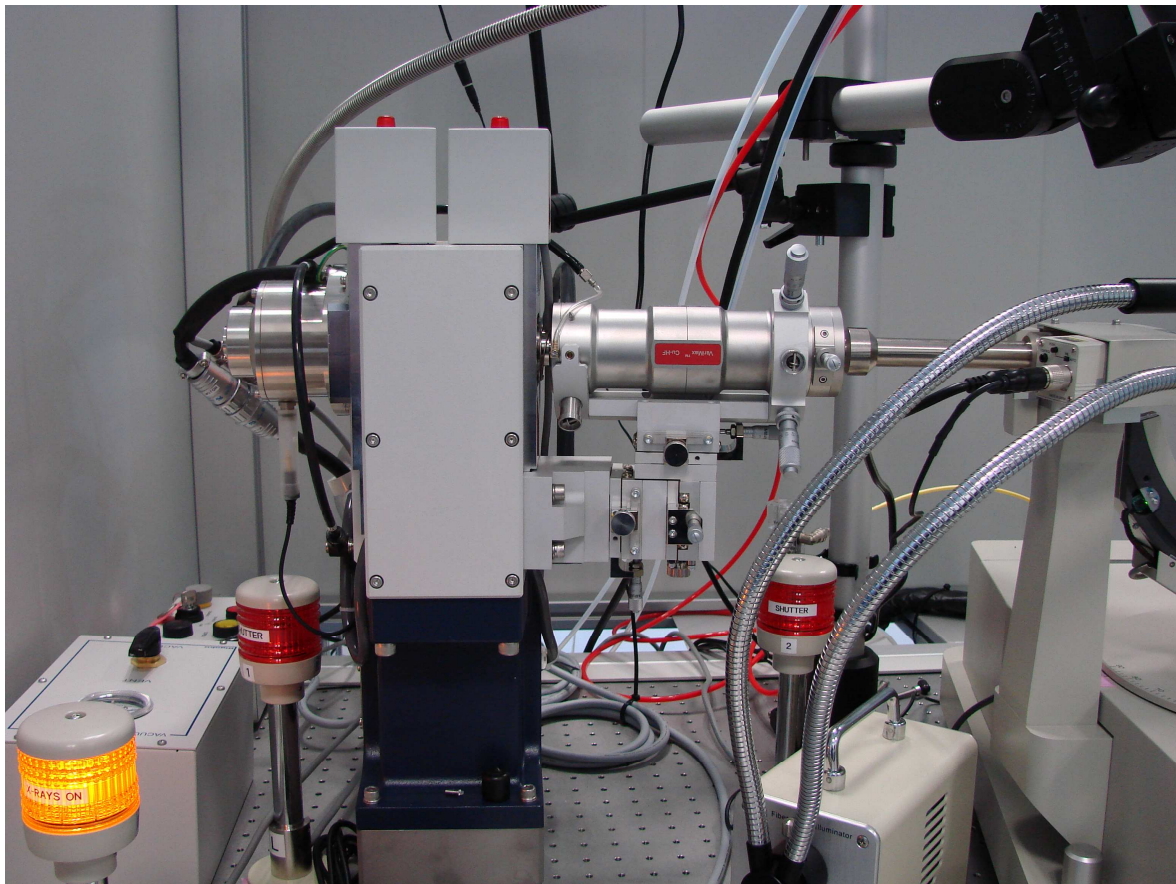
OPTYKA OGNISKUJĄCA WIĄZKĘ (Z POMPĄ PRÓŻNIOWĄ)
